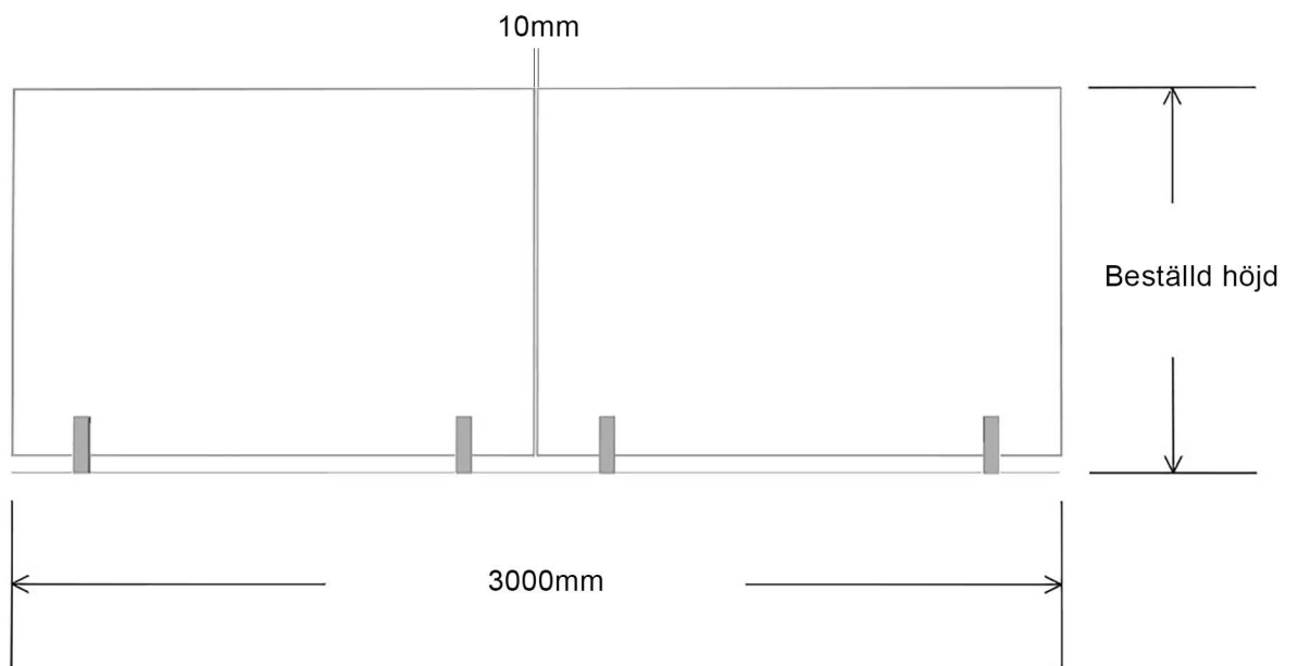
2st Arena golvbeslag - maxbredd glas 1500mm
